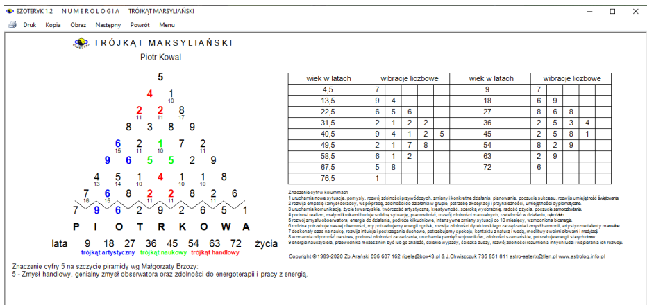
Rys.54. Trójkąt Marsyliński
