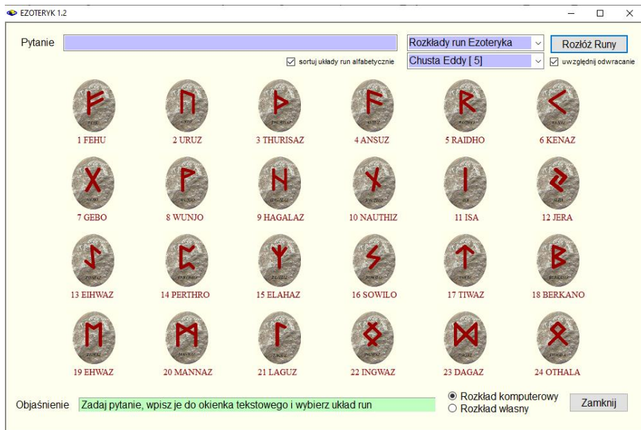
Rys.150. Futhark starszy.
